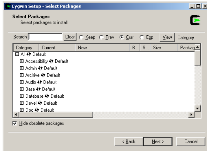
Abbildung 5: Cygwin – Packetauswahl
